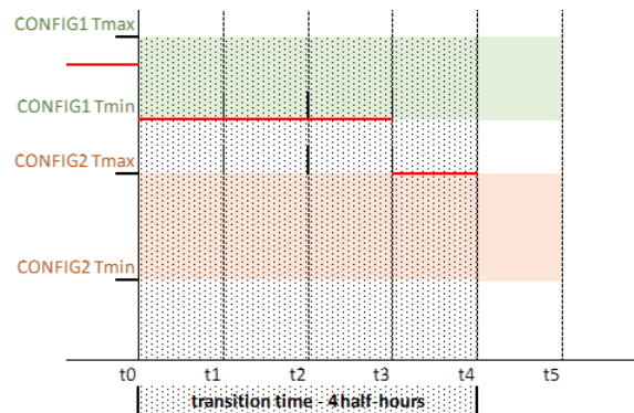
ΣΧΗΜΑ 31: ΜΕΤΑΒΑΣΗ ΣΕ ΚΑΤΩΤΕΡΗ ΔΙΑΤΑΞΗ ΛΕΙΤΟΥΡΓΙΑΣ ΧΩΡΙΣ ΝΑ ΥΠΑΡΧΕΙ ΕΠΙΚΑΛΥΨΗ ΤΩΝ ΟΡΙΩΝ ΛΕΙΤΟΥΡΓΙΑΣ
