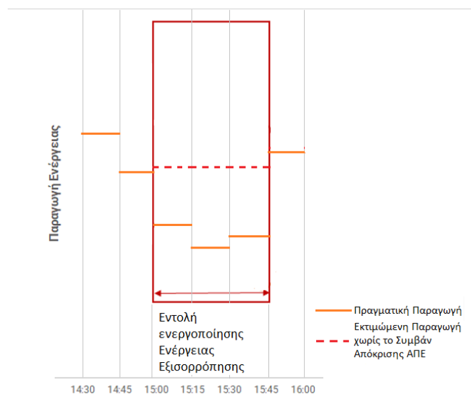
Σχήμα 5 Πραγματική και Εκτιμώμενη Παραγωγή σε Συμβάν Απόκρισης ΑΠΕ
