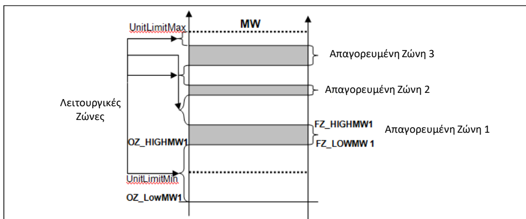
ΣΧΗΜΑ 28: ΑΠΑΓΟΡΕΥΜΕΝΗ ΖΩΝΗ ΣΤΙΣ ΚΑΤΑΝΕΜΟΜΕΝΕΣ ΥΔΡΟΗΛΕΚΤΡΙΚΕΣ ΜΟΝΑΔΕΣ ΠΑΡΑΓΩΓΗΣ
