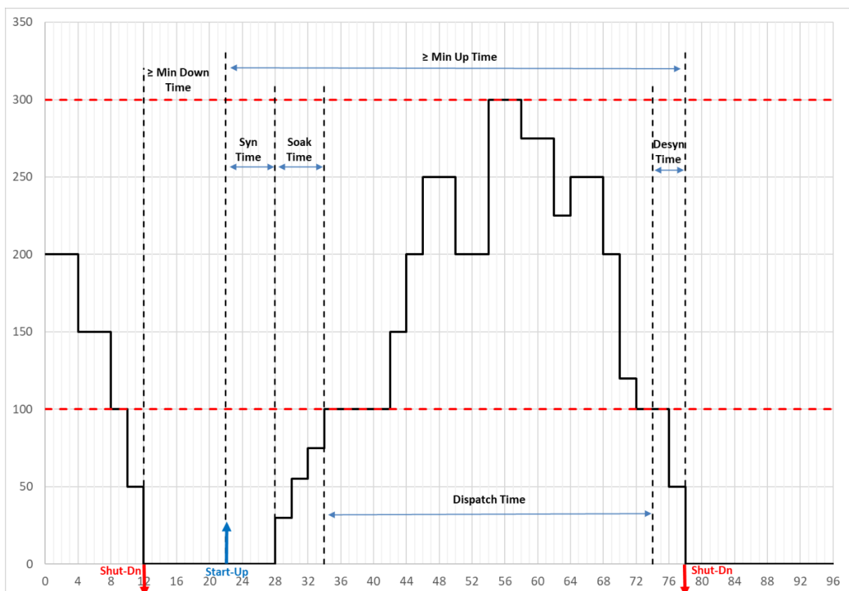
ΣΧΗΜΑ 20: ΜΟΝΤΕΛΟΠΟΙΗΣΗ ΤΗΣ ΔΙΑΔΙΚΑΣΙΑΣ ΕΚΚΙΝΗΣΗΣ - ΣΒΕΣΗΣ
