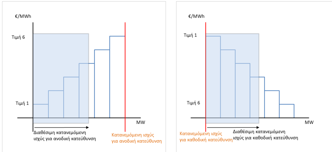
ΣΧΗΜΑ 13Γ ΒΗΜΑΤΙΚΕΣ ΠΡΟΣΦΟΡΕΣ ΑΝΟΔΙΚΗΣ (ΑΡΙΣΤΕΡΑ) ΚΑΙ ΚΑΘΟΔΙΚΗΣ (ΔΕΞΙΑ) ΕΝΕΡΓΕΙΑΣ ΕΞΙΣΟΡΡΟΠΗΣΗΣ ΓΙΑ ΚΑΤΑΝΕΜΟΜΕΝΕΣ ΟΝΤΟΤΗΤΕΣ ΑΠΟΘΗΚΕΥΣΗΣ
