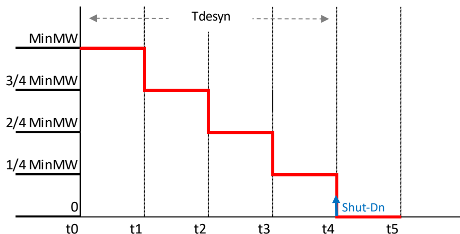
ΣΧΗΜΑ19: ΜΟΝΤΕΛΟΠΟΙΗΣΗ ΤΗΣ ΔΙΑΔΙΚΑΣΙΑΣ ΑΠΟΣΥΓΧΡΟΝΙΣΜΟΥ
