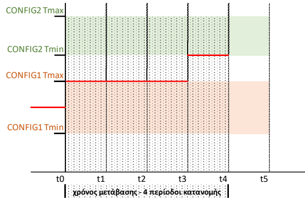
ΣΧΗΜΑ 29: ΜΕΤΑΒΑΣΗ ΣΕ ΑΝΩΤΕΡΗ ΔΙΑΤΑΞΗ ΛΕΙΤΟΥΡΓΙΑΣ ΧΩΡΙΣ ΝΑ ΥΠΑΡΧΕΙ ΕΠΙΚΑΛΥΨΗ ΤΩΝ ΟΡΙΩΝ ΛΕΙΤΟΥΡΓΙΑΣ
