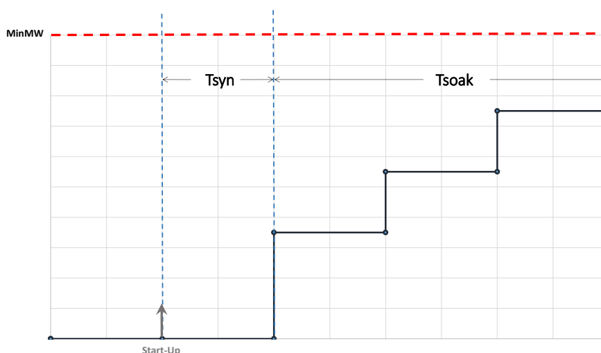
ΣΧΗΜΑ 18: ΕΚΚΙΝΗΣΗ ΜΟΝΑΔΑΣ ΠΑΡΑΓΩΓΗΣ
