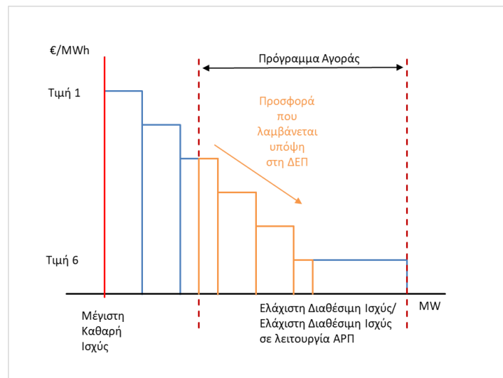
ΣΧΗΜΑ 17: ΚΑΘΟΔΙΚΗ ΠΡΟΣΦΟΡΑ ΕΝΕΡΓΕΙΑΣ ΕΞΙΣΟΡΡΟΠΗΣΗΣ ΜΙΑΣ ΟΝΤΟΤΗΤΑΣ ΥΠΗΡΕΣΙΩΝ ΕΞΙΣΟΡΡΟΠΗΣΗΣ
