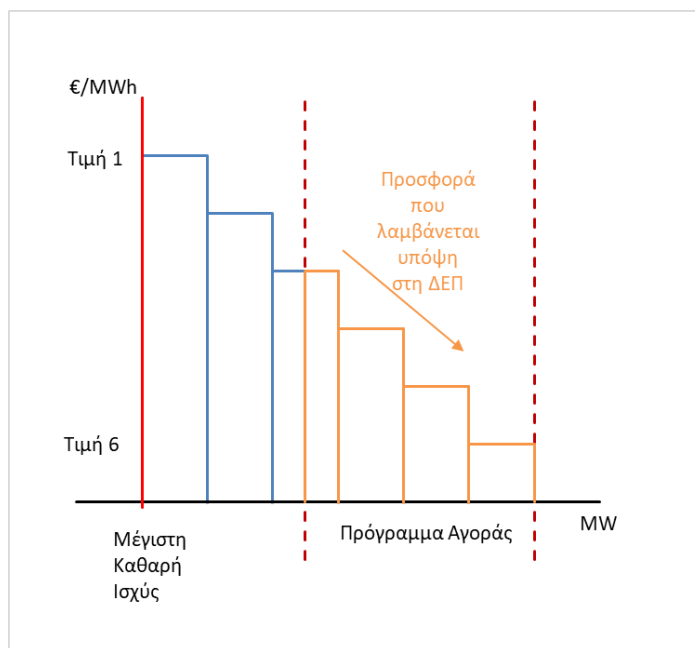
ΣΧΗΜΑ10: ΚΑΘΟΔΙΚΗ ΠΡΟΣΦΟΡΑ ΕΝΕΡΓΕΙΑΣ ΕΞΙΣΟΡΡΟΠΗΣΗΣ ΓΙΑ ΜΙΑ ΟΝΤΟΤΗΤΑ ΥΠΗΡΕΣΙΩΝ ΕΞΙΣΟΡΡΟΠΗΣΗΣ
