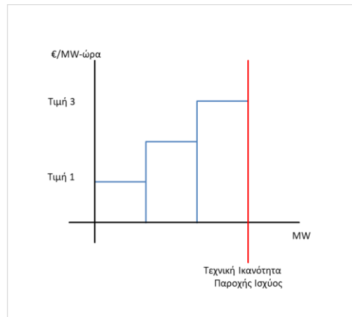
ΣΧΗΜΑ 15: ΜΟΡΦΗ ΠΡΟΣΦΟΡΑΣ ΑΝΟΔΙΚΗΣ ΚΑΙ ΚΑΘΟΔΙΚΗΣ ΙΣΧΥΟΣ ΕΞΙΣΟΡΡΟΠΗΣΗΣ
