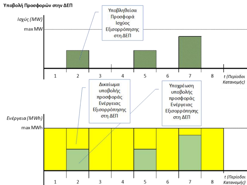
ΣΧΗΜΑ 8 ΠΑΡΑΔΕΙΓΜΑΤΑ ΥΠΟΒΟΛΗΣ ΠΡΟΣΦΟΡΩΝ ΙΣΧΥΟΣ & ΕΝΕΡΓΕΙΑΣ ΕΞΙΣΟΡΡΟΠΗΣΗΣ ΣΤΗ ΔΕΠ ΓΙΑ ΚΑΤΑΝΕΜΟΜΕΝΕΣ ΟΝΤΟΤΗΤΕΣ ΑΠΟΘΗΚΕΥΣΗΣ, ΚΑΤΑΝΕΜΟΜΕΝΑ ΧΑΡΤΟΦΥΛΑΚΙΑ ΕΛΕΓΧΟΜΕΝΗΣ / ΜΗ ΕΛΕΓΧΟΜΕΝΗΣ ΠΑΡΑΓΩΓΗΣ ΚΑΙ ΧΑΡΤΟΦΥΛΑΚΙΑ ΚΑΤΑΝΕΜΟΜΕΝΟΥ ΦΟΡΤΙΟΥ
