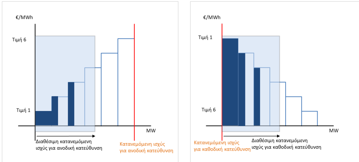
ΣΧΗΜΑ 13Α ΠΑΡΑΔΕΙΓΜΑΤΑ ΒΗΜΑΤΙΚΩΝ ΠΡΟΣΦΟΡΩΝ ΑΝΟΔΙΚΗΣ (ΑΡΙΣΤΕΡΑ) ΚΑΙ ΚΑΘΟΔΙΚΗΣ (ΔΕΞΙΑ) ΕΝΕΡΓΕΙΑΣ ΕΞΙΣΟΡΡΟΠΗΣΗΣ ΓΙΑ ΧΑΡΤΟΦΥΛΑΚΙΑ ΚΑΤΑΝΕΜΟΜΕΝΟΥ ΦΟΡΤΙΟΥ
