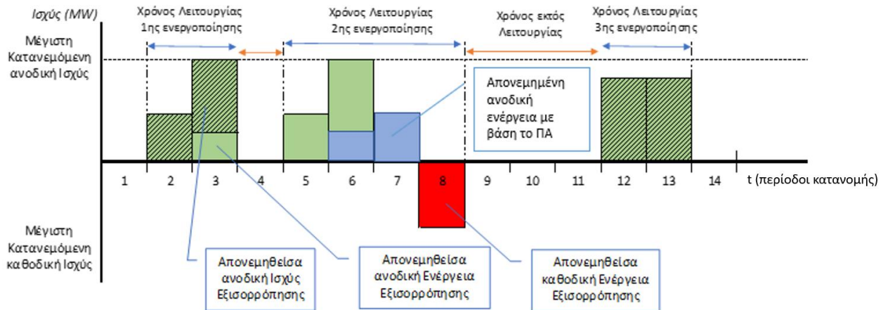
ΣΧΗΜΑ 21: ΚΥΚΛΟΙ ΕΝΕΡΓΟΠΟΙΗΣΕΩΝ ΓΙΑ ΤΗΝ ΠΑΡΟΧΗ ΕΝΕΡΓΕΙΑΣ Η/ΚΑΙ ΙΣΧΥΟΣ ΕΞΙΣΟΡΡΟΠΗΣΗΣ
