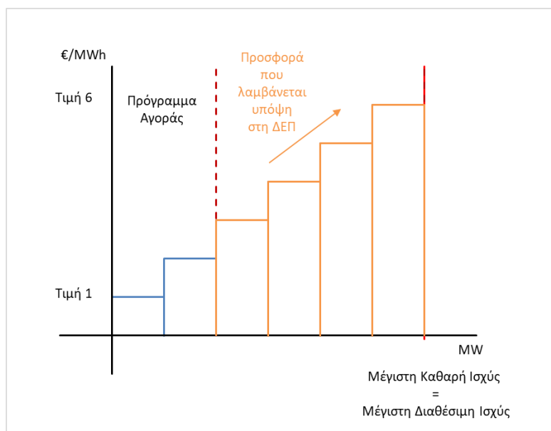
ΣΧΗΜΑ 9: ΑΝΟΔΙΚΗ ΠΡΟΣΦΟΡΑ ΕΝΕΡΓΕΙΑΣ ΕΞΙΣΟΡΡΟΠΗΣΗΣ ΓΙΑ ΜΙΑ ΟΝΤΟΤΗΤΑ ΥΠΗΡΕΣΙΩΝ ΕΞΙΣΟΡΡΟΠΗΣΗΣ ΟΤΑΝ ΔΕΝ ΕΙΝΑΙ ΠΛΗΡΩΣ ΔΙΑΘΕΣΙΜΗ (ΕΠΑΝΩ) ΚΑΙ ΟΤΑΝ ΕΙΝΑΙ ΠΛΗΡΩΣ ΔΙΑΘΕΣΙΜΗ (ΚΑΤΩ)
