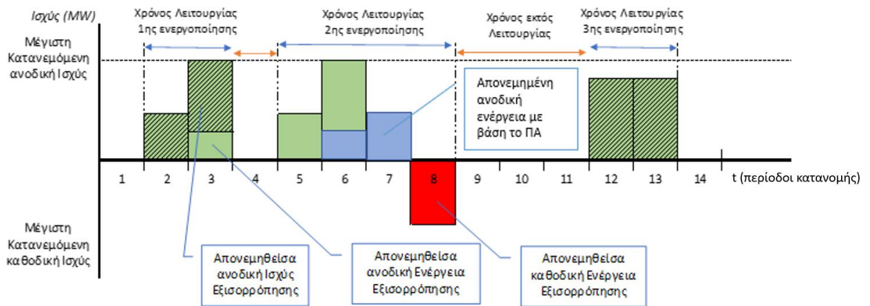
ΣΧΗΜΑ 4: ΚΥΚΛΟΙ ΕΝΕΡΓΟΠΟΙΗΣΕΩΝ ΓΙΑ ΤΗΝ ΠΑΡΟΧΗ ΕΝΕΡΓΕΙΑΣ Η/ΚΑΙ ΙΣΧΥΟΣ ΕΞΙΣΟΡΡΟΠΗΣΗΣ
