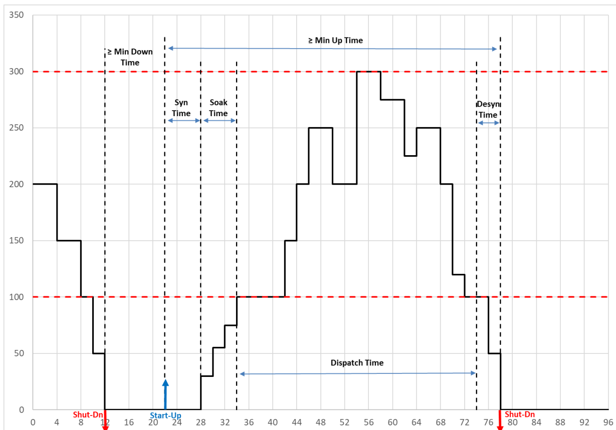
ΣΧΗΜΑ 3: ΜΟΝΤΕΛΟ ΕΚΚΙΝΗΣΗΣ ΚΑΙ ΣΒΕΣΗΣ
