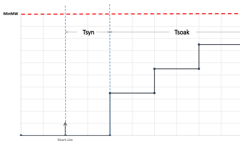
ΣΧΗΜΑ 1: ΕΚΚΙΝΗΣΗ ΜΟΝΑΔΑΣ ΠΑΡΑΓΩΓΗΣ
