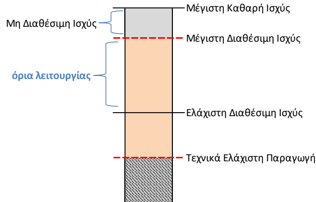
ΣΧΗΜΑ 6: ΟΡΙΑ ΛΕΙΤΟΥΡΓΙΑΣ ΚΑΤΑΝΕΜΟΜΕΝΩΝ ΧΑΡΤΟΦΥΛΑΚΙΩΝ ΕΛΕΓΧΟΜΕΝΗΣ ΠΑΡΑΓΩΓΗΣ
