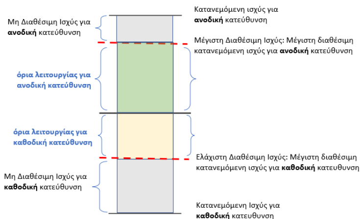
ΣΧΗΜΑ 7: ΟΡΙΑ ΛΕΙΤΟΥΡΓΙΑΣ ΚΑΤΑΝΕΜΟΜΕΝΩΝ ΧΑΡΤΟΦΥΛΑΚΙΩΝ ΜΗ ΕΛΕΓΧΟΜΕΝΗΣ ΠΑΡΑΓΩΓΗΣ, ΧΑΡΤΟΦΥΛΑΚΙΩΝ ΚΑΤΑΝΕΜΟΜΕΝΟΥ ΦΟΡΤΙΟΥ ΚΑΙ ΚΑΤΑΝΕΜΟΜΕΝΩΝ ΟΝΤΟΤΗΤΩΝ ΑΠΟΘΗΚΕΥΣΗΣ
