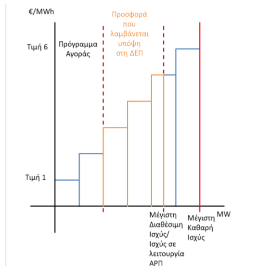
ΣΧΗΜΑ 16: ΑΝΟΔΙΚΗ ΠΡΟΣΦΟΡΑ ΕΝΕΡΓΕΙΑΣ ΕΞΙΣΟΡΡΟΠΗΣΗΣ ΜΙΑΣ ΟΝΤΟΤΗΤΑΣ ΥΠΗΡΕΣΙΩΝ ΕΞΙΣΟΡΡΟΠΗΣΗΣ
