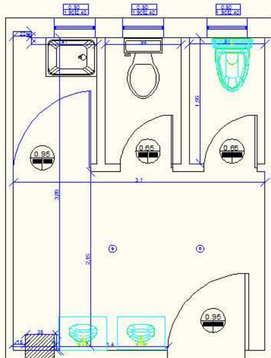
ΚΑΤΟΨΗ ΝΕΟΥ WC ΤΗΛΕΠΙΚΟΙΝΩΝΙΕΣ
