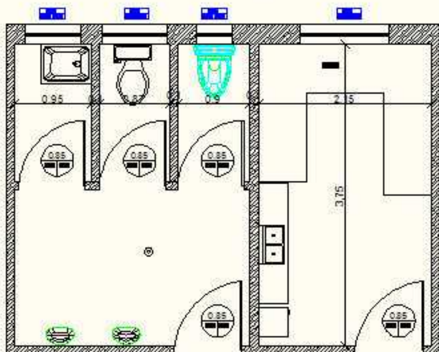
ΚΑΤΟΨΗ ΝΕΟ ΨΟ ΚΤΙΡΙΟΥ ΠΡΟΣΤΑΣΙΑΣ
