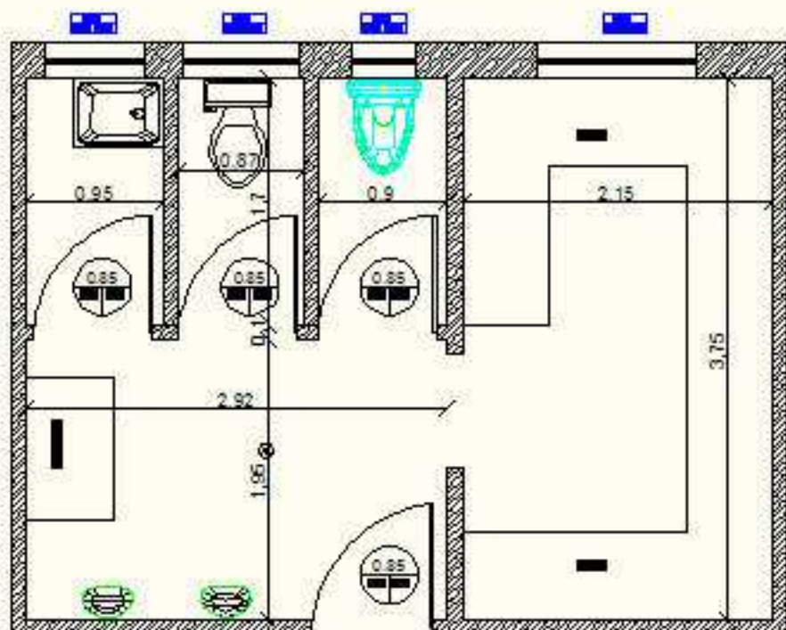
ΚΑΤΟΧΗ ΥΠΑΡΧΟΝ ΩΣ ΚΤΙΡΙΟΥ ΠΡΟΣΤΑΣΙΑΣ
