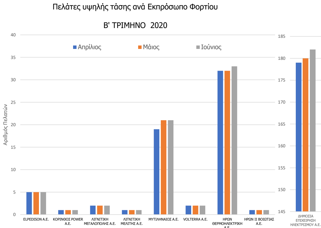
Γράφημα 2.2: Αριθμός των πελατών υψηλής τάσης ανά Εκπρόσωπο Φορτίου
