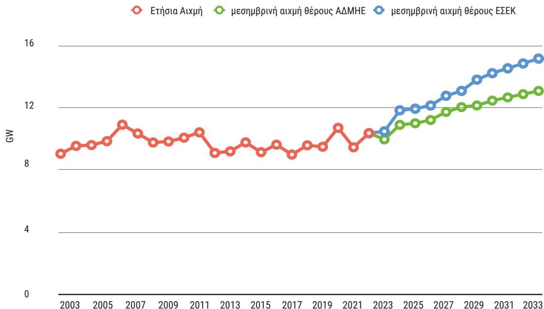
Γράφημα 3.6 Εξέλιξη και πρόβλεψη ετήσιας αιχμής φορτίου έως το 2034
