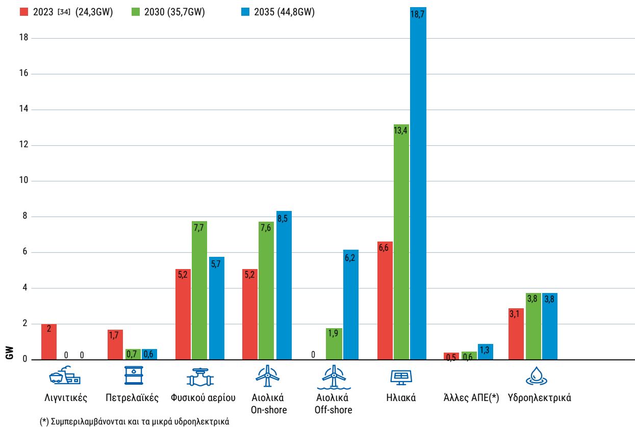
Γράφημα 3.2 Βασικά χαρακτηριστικά του συστήματος ηλεκτροπαραγωγής μέχρι το έτος 2035 (πηγή προσχέδιο αναθεωρημένου ΕΣΕΚ)
