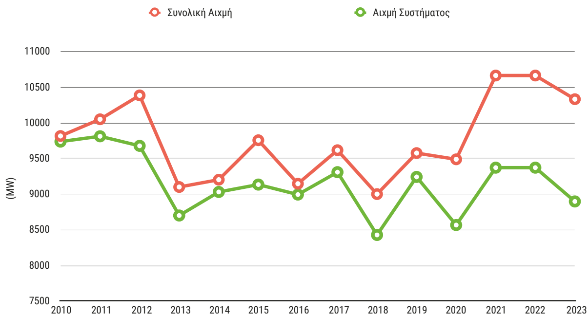
Γράφημα 3.7 Επίδραση διεσπαρμένης παραγωγής στην αιχμή φορτίου
