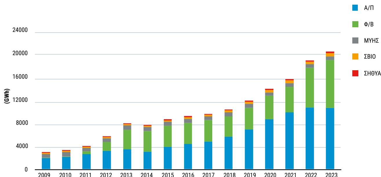
Γράφημα 4.4 Παραγωγή της ηλεκτρικής ενέργειας από Σταθμούς Παραγωγής ΑΠΕ και ΣΗΘΥΑ στο Διασυνδεδεμένο Σύστημα (GWh)
