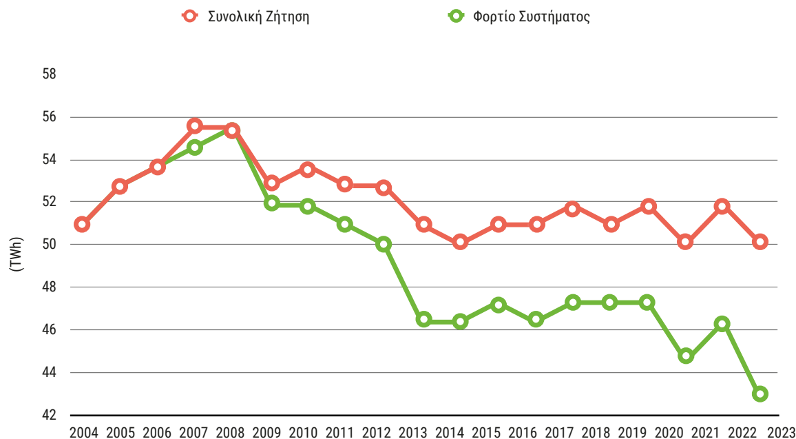
Γράφημα 3.5 Επίδραση Διεσπαρμένης Παραγωγής στη ζήτηση της ηλεκτρικής ενέργειας
