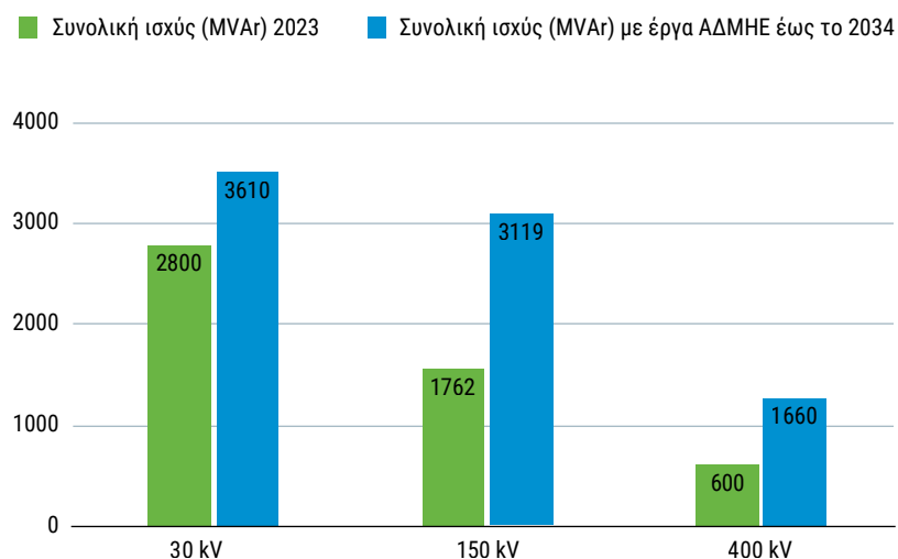
Γράφημα 3.10 Συνολική ισχύς αυτεπαγωγών για αντιστάθμιση άεργου ισχύος
