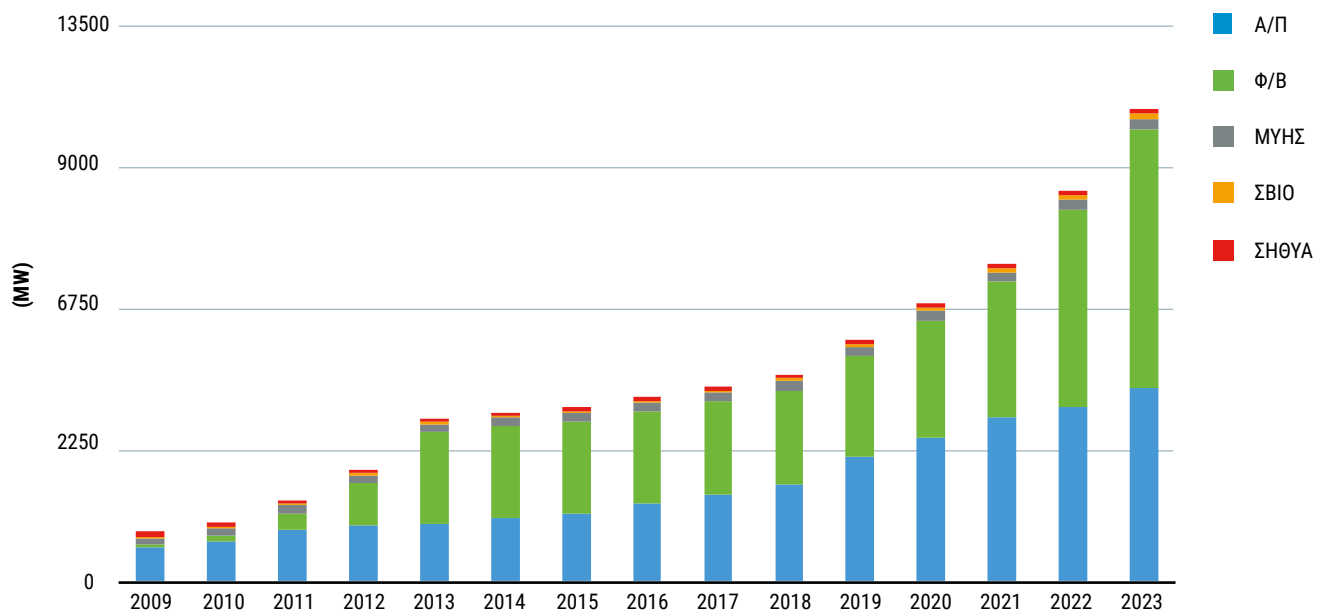
Γράφημα 4.5 Εγκατεστημένη ισχύς Σταθμών Παραγωγής ΑΠΕ και ΣΗΘΥΑ στο Διασυνδεδεμένο Σύστημα (MW) [49]
