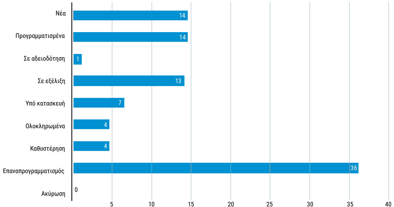
Γράφημα 6.1 Έργα Ανάπτυξης Συστήματος Μεταφοράς στο ΔΠΑ 2025-2034
