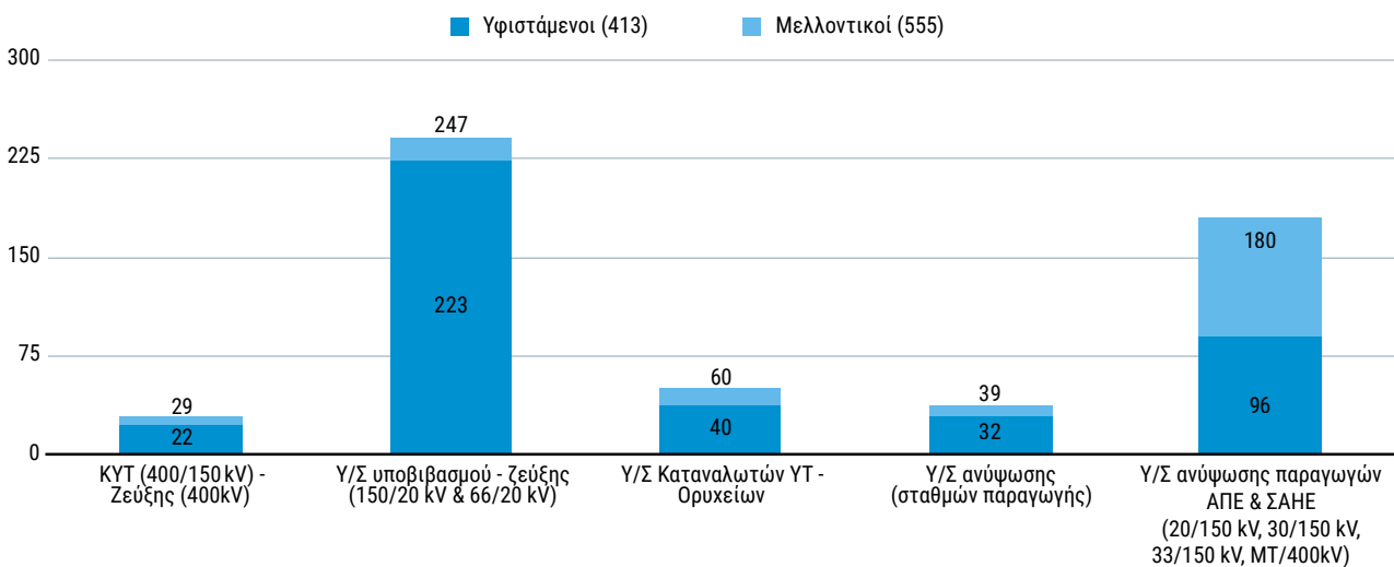
Γράφημα 3.8 Υποσταθμοί και Κέντρα Υπερυψηλής Τάσης (ΚΥΤ) [38]
