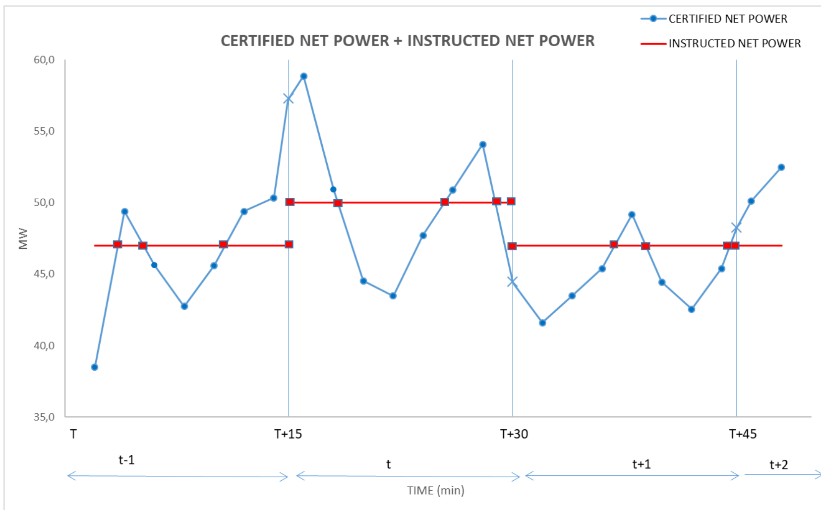
ΔΙΑΓΡΑΜΜΑ 11: ΠΙΣΤΟΠΟΙΗΜΕΝΗ ΚΑΘΑΡΗ ΙΣΧΥΣ (ΜΠΛΕ ΚΑΜΠΥΛΗ) ΚΑΙ ΕΠΙΒΕΒΑΗΜΕΝΗ ΜΕΣΗ ΙΣΧΥΣ (ΚΟΚΚΙΝΗ ΚΑΜΠΥΛΗ)
