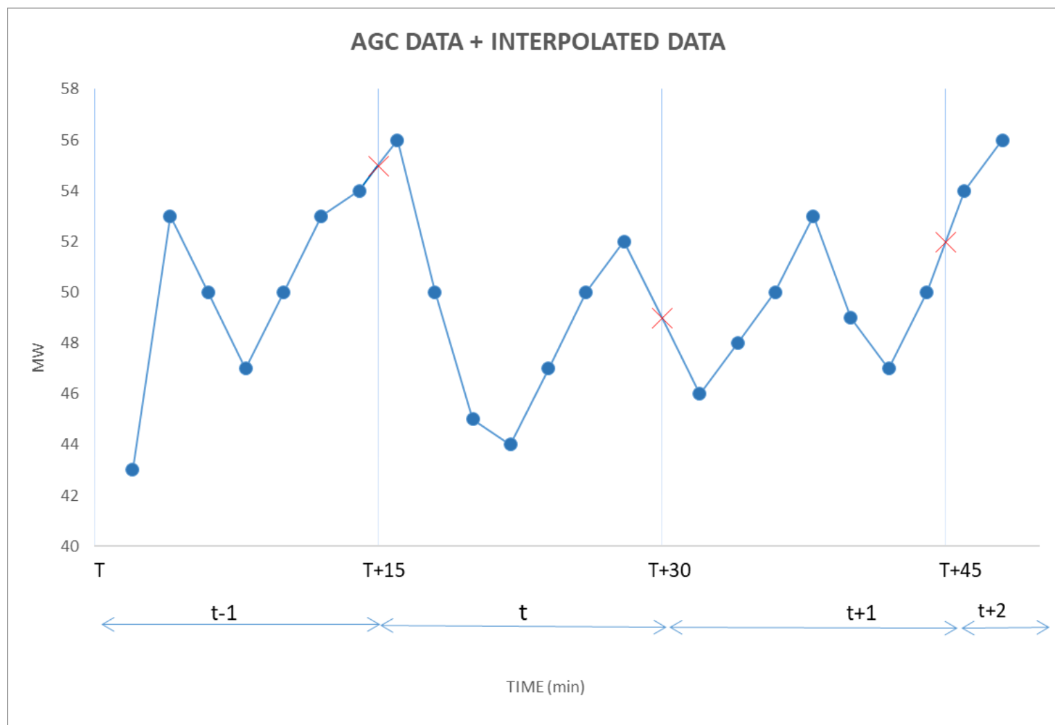
ΔΙΑΓΡΑΜΜΑ 5: ΕΚΤΙΜΗΣΗ ΜΙΚΤΗΣ ΙΣΧΥΟΣ ΣΤΑ ΣΗΜΕΙΑ ΤΗΣ ΑΡΧΗΣ ΚΑΘΕ ΠΕΡΙΟΔΟΥ ΕΚΚΑΘΑΡΙΣΗΣ ΑΠΟΚΑΙΣΕΩΝ ΜΕ ΤΗΝ ΧΡΗΣΗ ΓΡΑΜΜΙΚΗΣ ΠΑΡΕΜΒΟΛΗΣ
