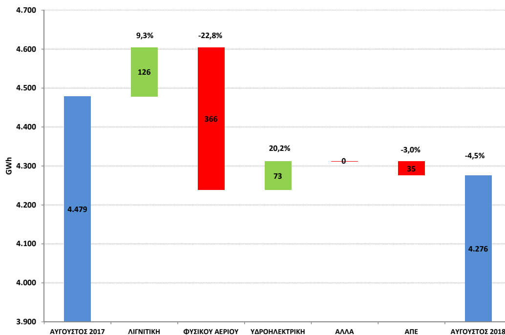
ΜΕΤΑΒΟΛΗ ΠΑΡΑΓΩΓΗΣ ΑΥΓΟΥΣΤΟΥ 2017 ΕΝΑΝΤΙ ΑΥΓΟΥΣΤΟΥ 2018 (GWh)
