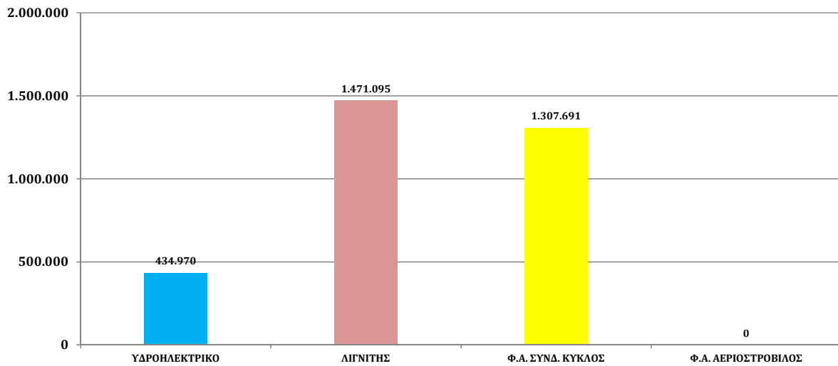
ΚΑΘΑΡΗ ΠΑΡΑΓΩΓΗ (MWh) - ΑΥΓΟΥΣΤΟΣ 2018
