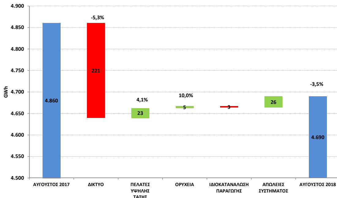
ΜΕΤΑΒΟΛΗ ΖΗΤΗΣΗΣ ΑΥΓΟΥΣΤΟΥ 2017 ΕΝΑΝΤΙ ΑΥΓΟΥΣΤΟΥ 2018
