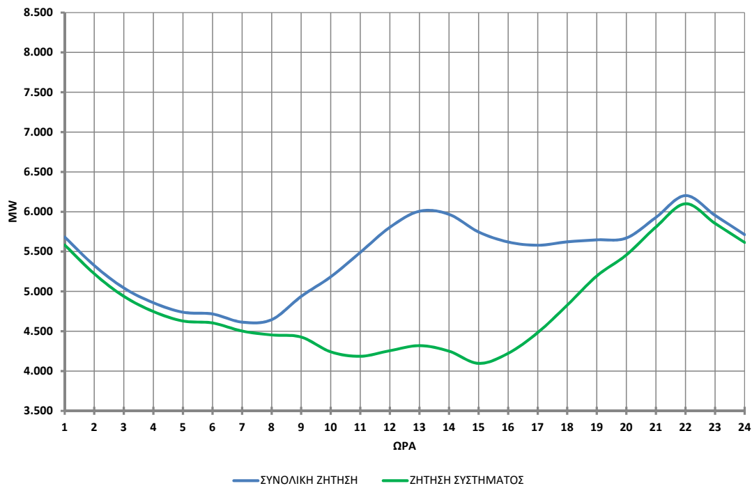
ΩΡΙΑΙΑ ΖΗΤΗΣΗ ΚΑΤΑ ΤΗΝ ΗΜΕΡΑ ΣΥΝΟΛΙΚΟΥ ΕΛΑΧΙΣΤΟΥ ΤΟΥ ΜΗΝΑ: 15/8/2018
