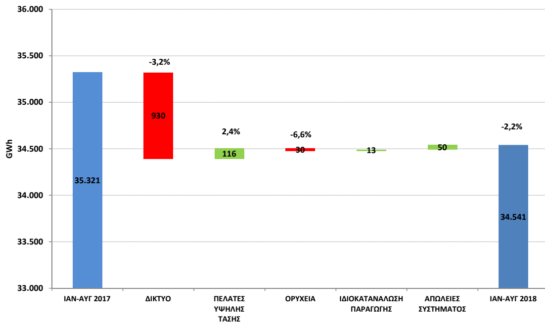
ΜΕΤΑΒΟΛΗ ΖΗΤΗΣΗΣ ΙΑΝΟΥΑΡΙΟΥ-ΑΥΓΟΥΣΤΟΥ 2017 ΕΝΑΝΤΙ ΙΑΝΟΥΑΡΙΟΥ-ΑΥΓΟΥΣΤΟΥ 2018
