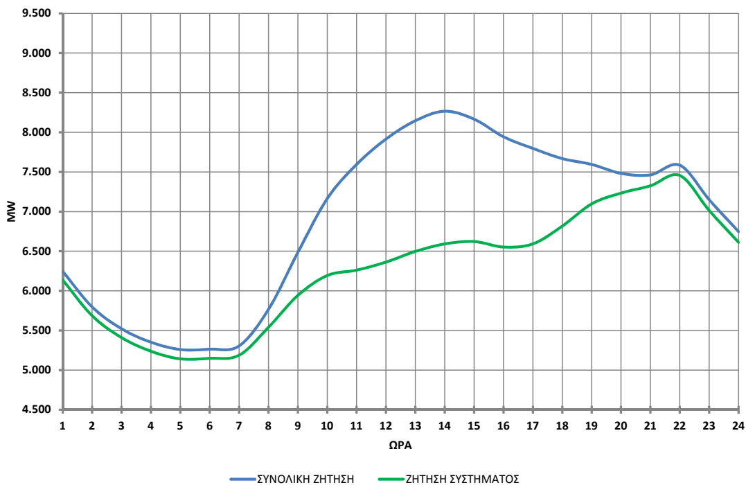
ΩΡΙΑΙΑ ΖΗΤΗΣΗ ΚΑΤΑ ΤΗΝ ΗΜΕΡΑ ΣΥΝΟΛΙΚΟΥ ΜΕΓΙΣΤΟΥ ΤΟΥ ΜΗΝΑ: 2/8/2018
