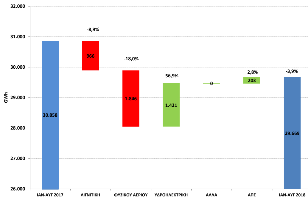
ΜΕΤΑΒΟΛΗ ΠΑΡΑΓΩΓΗΣ ΙΑΝΟΥΑΡΙΟΥ-ΑΥΓΟΥΣΤΟΥ 2017 ΕΝΑΝΤΙ ΙΑΝΟΥΑΡΙΟΥ-ΑΥΓΟΥΣΤΟΥ 2018 (GWh)
