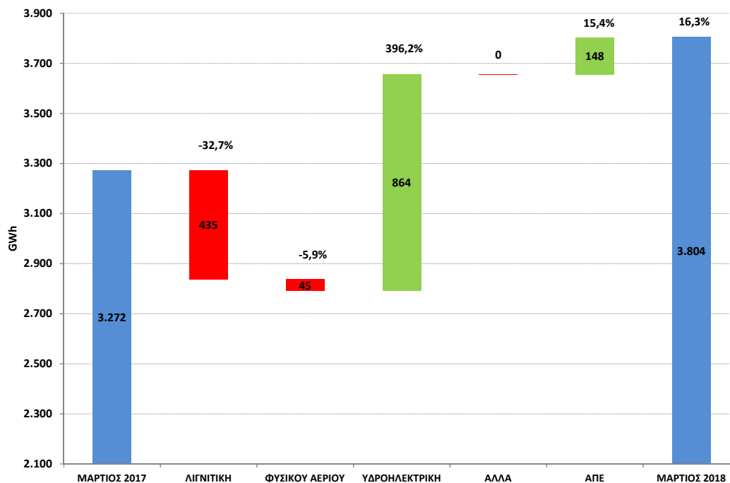
ΜΕΤΑΒΟΛΗ ΠΑΡΑΓΩΓΗΣ ΜΑΡΤΙΟΥ 2017 ΕΝΑΝΤΙ ΜΑΡΤΙΟΥ 2018 (GWh)
