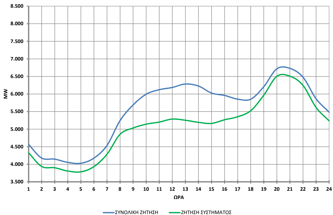
ΩΡΙΑΙΑ ΖΗΤΗΣΗ ΚΑΤΑ ΤΗΝ ΗΜΕΡΑ ΣΥΝΟΛΙΚΟΥ ΕΛΑΧΙΣΤΟΥ ΤΟΥ ΜΗΝΑ: 19/3/2018
