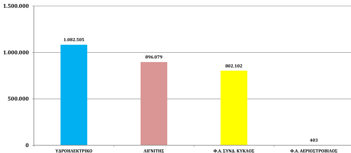
ΚΑΘΑΡΗ ΠΑΡΑΓΩΓΗ (MWh) - ΜΑΡΤΙΟΣ 2018
