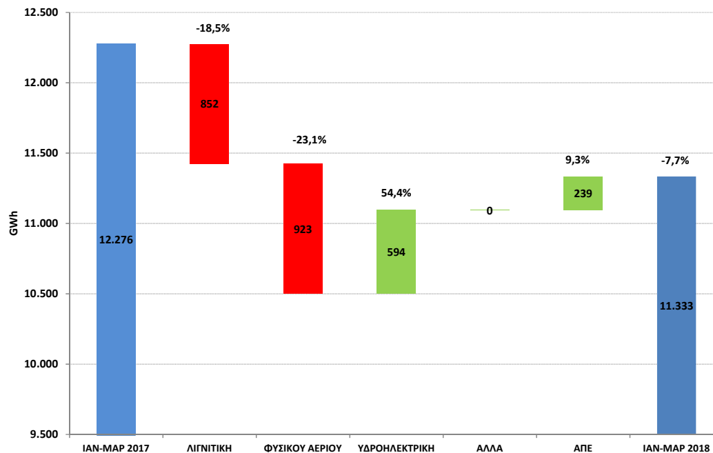
ΜΕΤΑΒΟΛΗ ΠΑΡΑΓΩΓΗΣ ΙΑΝΟΥΑΡΙΟΥ-ΜΑΡΤΙΟΥ 2017 ΕΝΑΝΤΙ ΙΑΝΟΥΑΡΙΟΥ-ΜΑΡΤΙΟΥ 2018 (GWh)
