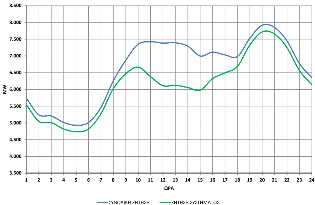
ΩΡΙΑΙΑ ΖΗΤΗΣΗ ΚΑΤΑ ΤΗΝ ΗΜΕΡΑ ΣΥΝΟΛΙΚΟΥ ΜΕΓΙΣΤΟΥ ΤΟΥ ΜΗΝΑ: 1/3/2018
