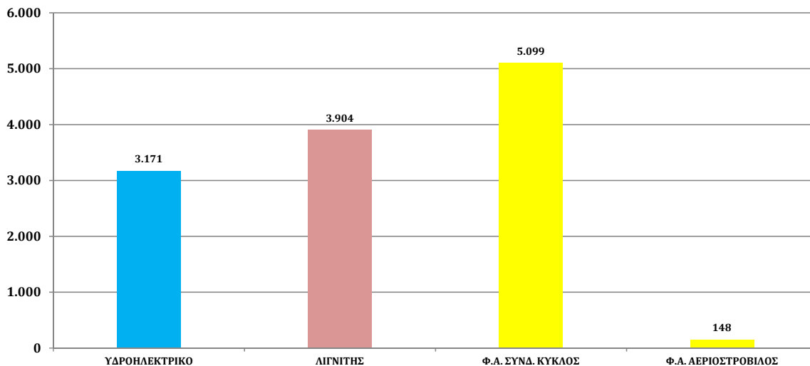
ΚΑΘΑΡΗ ΙΣΧΥΣ (MW) - ΜΑΡΤΙΟΣ 2018
