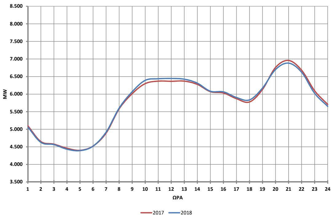
ΜΕΣΗ ΩΡΙΑΙΑ ΣΥΝΟΛΙΚΗ ΖΗΤΗΣΗ ΕΡΓΑΣΙΜΩΝ ΗΜΕΡΩΝ ΤΟΥ ΜΗΝΑ ΜΑΡΤΙΟΥ
