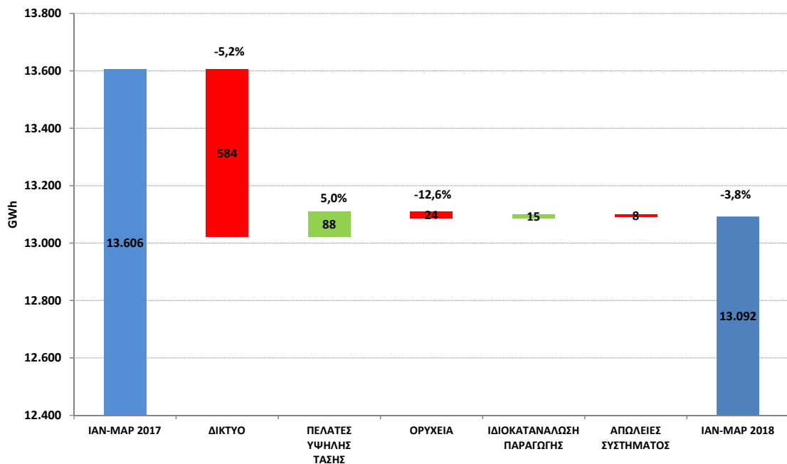
ΜΕΤΑΒΟΛΗ ΖΗΤΗΣΗΣ ΙΑΝΟΥΑΡΙΟΥ-ΜΑΡΤΙΟΥ 2017 ΕΝΑΝΤΙ ΙΑΝΟΥΑΡΙΟΥ-ΜΑΡΤΙΟΥ 2018
