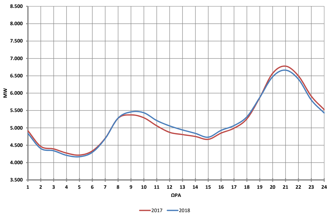
ΜΕΣΗ ΩΡΙΑΙΑ ΖΗΤΗΣΗ ΣΥΣΤΗΜΑΤΟΣ ΕΡΓΑΣΙΜΩΝ ΗΜΕΡΩΝ ΤΟΥ ΜΗΝΑ ΜΑΡΤΙΟΥ
